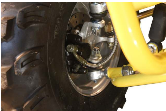
Передний тормоз
